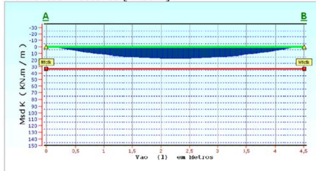
Momentos Flectores [ MsdK ]
