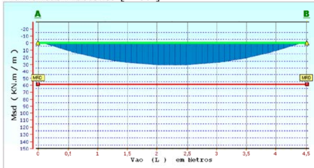
Momentos Flectores [ Msd ]
