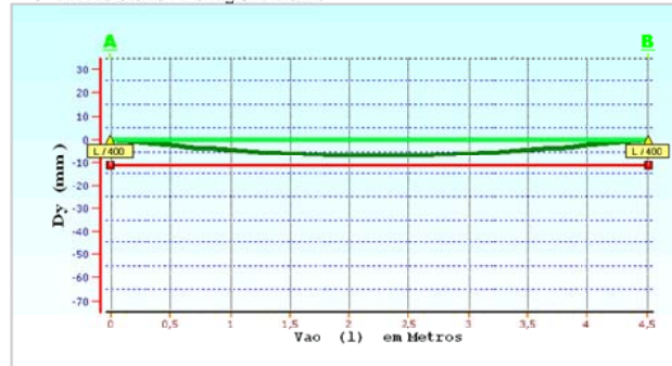
Deformada a Longo Prazo
