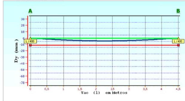
Deformada a Curto Prazo
