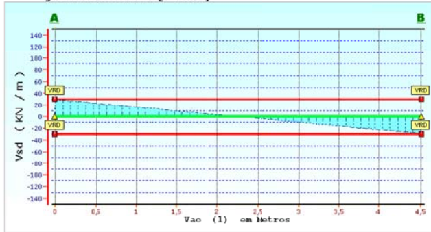
Esforço Transverso [ Vsd ]
