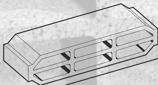
BLOCO 65X15X21.5
