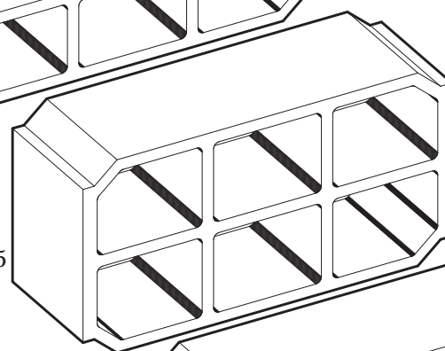
BLOCO 65X34X21.5
