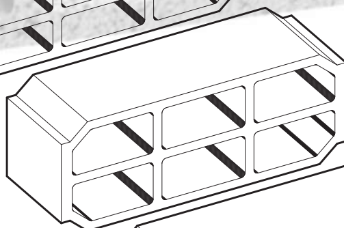
BLOCO 65X25X21.5
